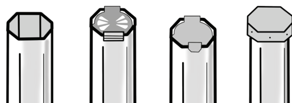
Non obturé DANGEREUX Obturé plastique DANGEREUX Obturé métal INOFFENSIF Obturé en usine INOFFENSIF
